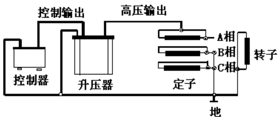
图 9 测量定子的某相连线图
