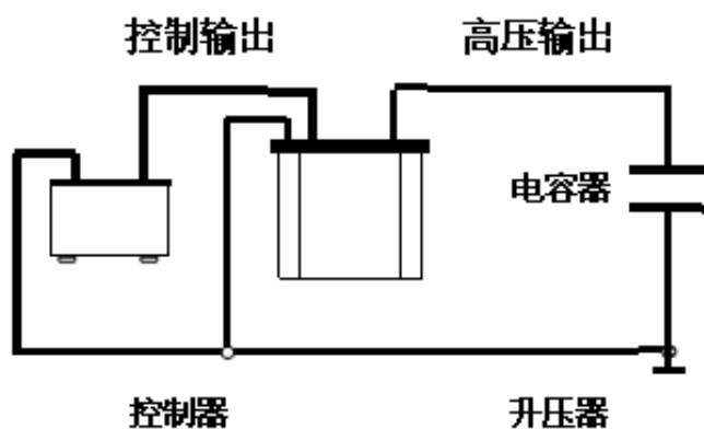
图 10 测量电容器的连线图
