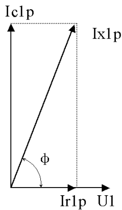
图 8 投影法
