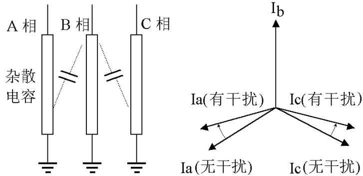
图 9、一字排列避雷器的相间干扰
